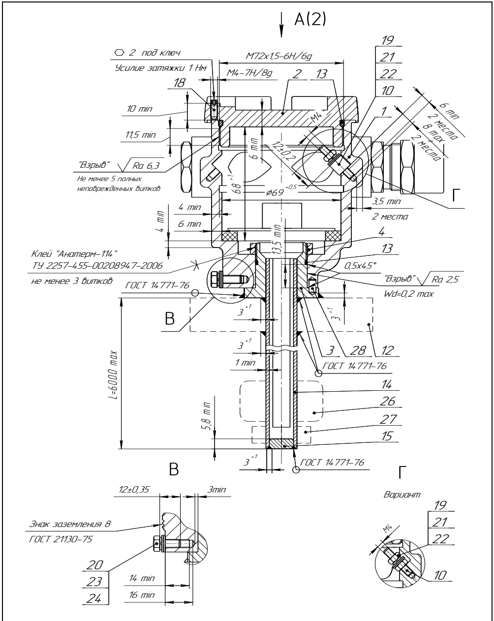
Рисунок 11 (лист 1 из 5) – Чертеж средств взрывозащиты
