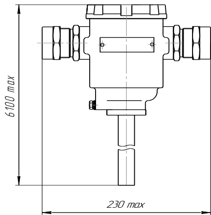
Рисунок 11 (лист 3 из 5) – Чертеж средств взрывозащиты
