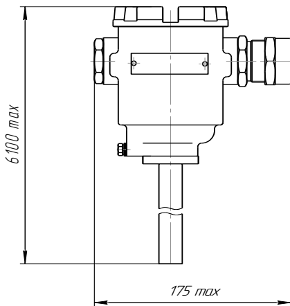
Рисунок 11 (лист 3 из 5) – Чертеж средств взрывозащиты
