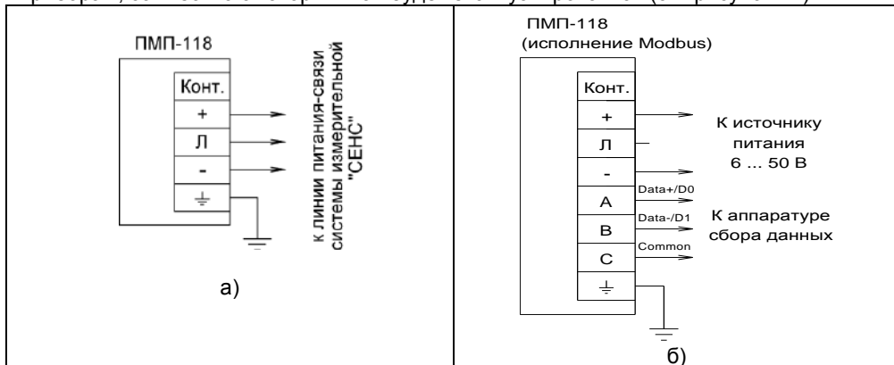
Рисунок 12 – Схема подключения: а) к системе с протоколом СЕНС; б) к системе с протоколом Modbus
